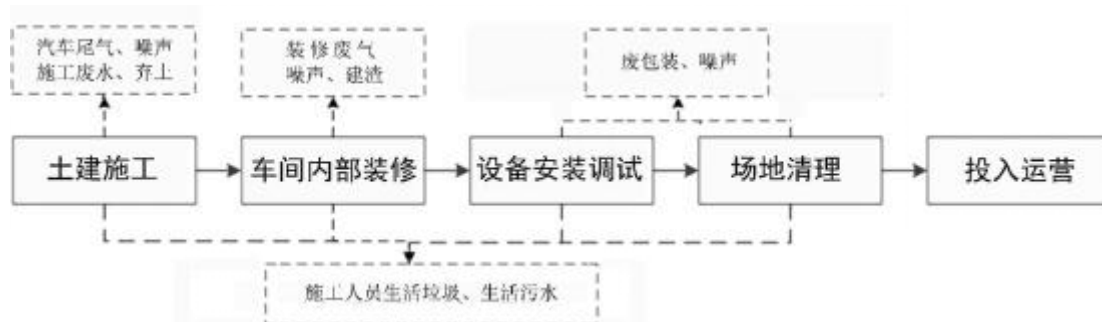
图 3-1 施工期工艺流程及产污环节示意图
